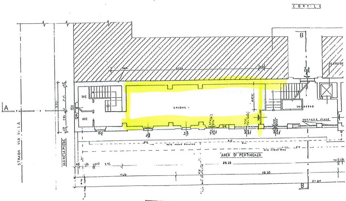
PIANTA PIANO TERRA VERSANTE NORD
