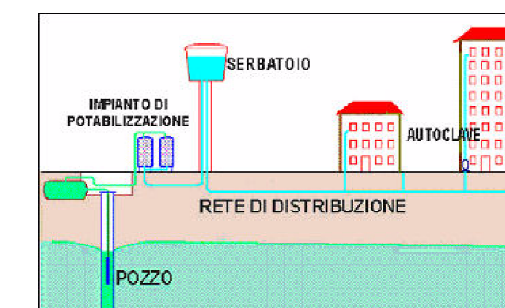
Rete dell'Acquedotto
