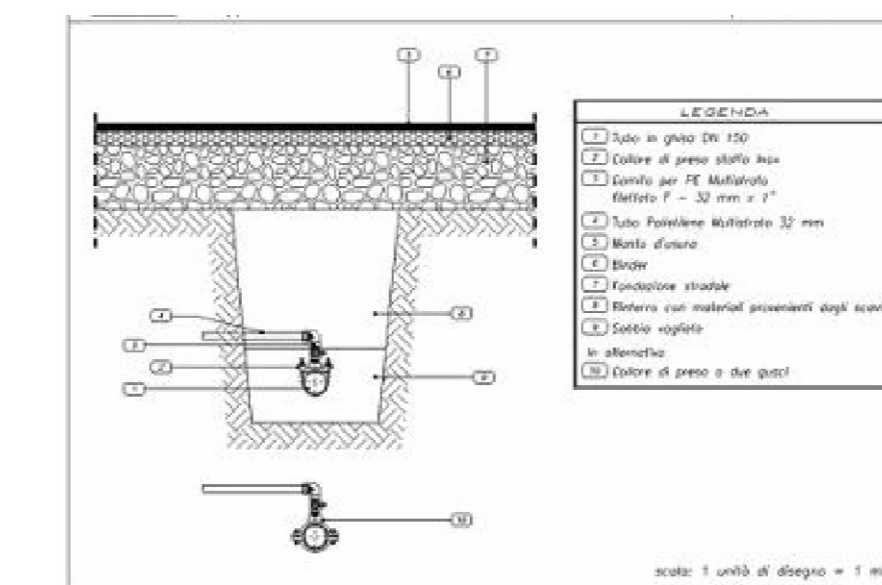
Allaccio Acquedotto
