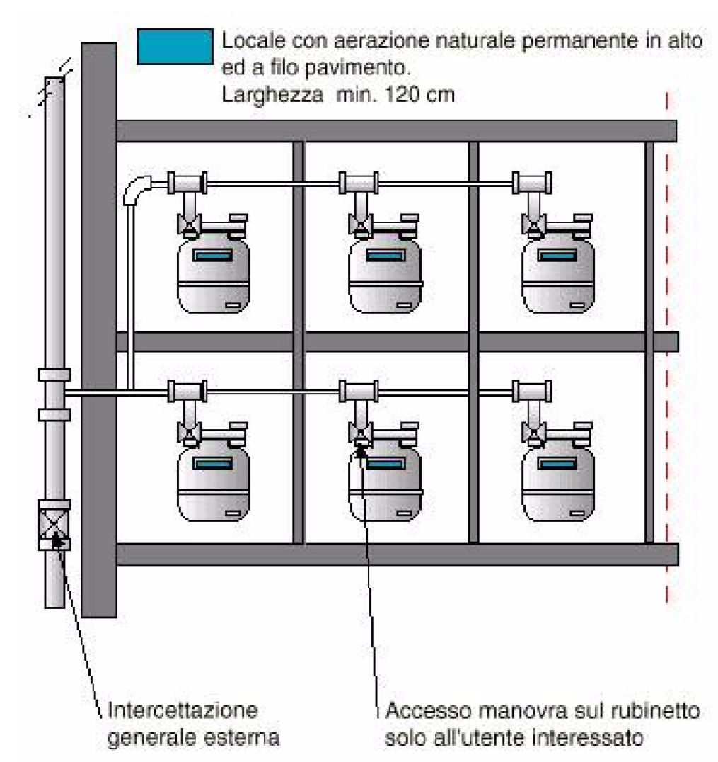
Contatori Multiutenza
