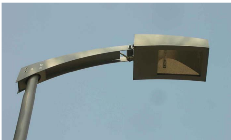
Via XXV Aprile: proiettore per l'illuminazione stradale dotato di vetro di chiusura piano, sorgente ai vapori di sodio ad alta pressione ed orientamento conformi alle vigenti leggi regionali.
